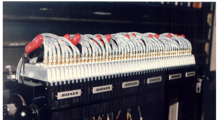
Schneidkassette für Schnittbreiten ab 6 mm
